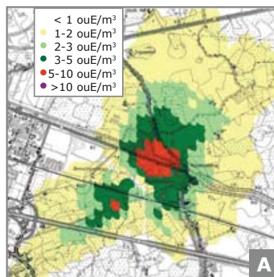
A Einfluss Geruch auf die Umgebung
